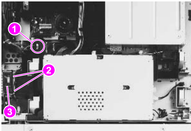
Power-supply fan
