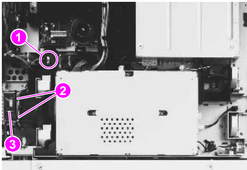
Power-supply fan
